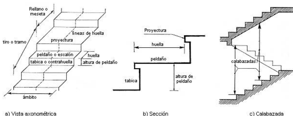
Fig. 1: Representación de las partes de una escalera
