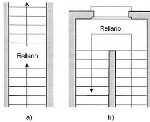
Fig 2: Escalera recta de uno y dos tramos
