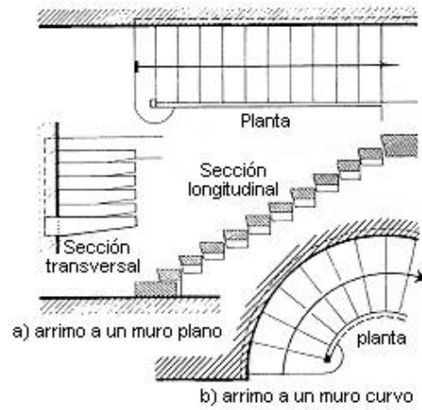
Fig 5: Escalera de arrimo o adosada
