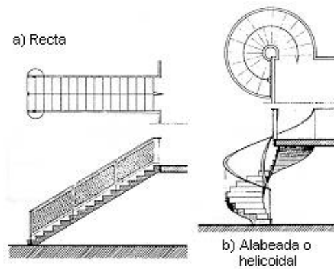
Fig 6: Escalera de suelo a suelo
