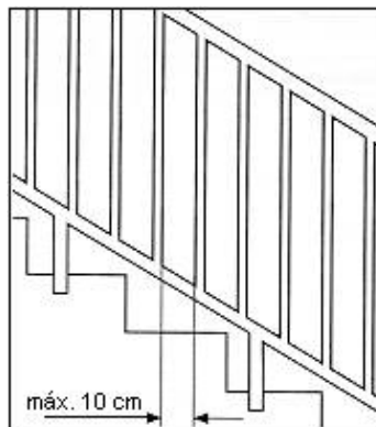
Fig. 12: Barandilla protegida con barras verticales de separación máxima 10 cm
