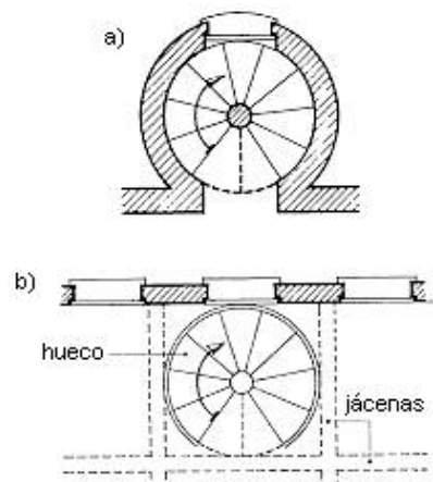
Fig 4: Escalera de tiro curvo o caracol
